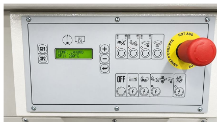
ДИСПЛЕЙ ЗА ТЕМПЕРАТУРА, ИЗБОР НА АГРЕГАТИТЕ С LED БУТОНИ И АВАРИЙНО СПИРАНЕ
