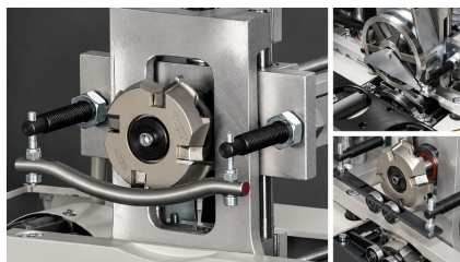
ФРЕЗОВАНЕ НА НИВОТО ОТГОРЕ / ОТДОЛУ С ФРЕЗИ Z4 ОТ 75 ММ И ДИСКОВИ КОПИРИ
